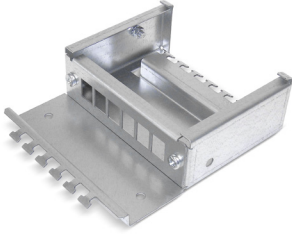
Base de la caja con placa frontal montada 6x MGK (entrega sin placa frontal)
