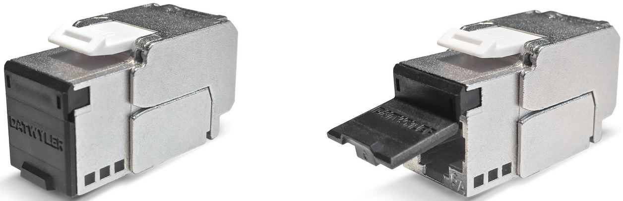
RJ45-Modul KS-TC Plus Cat.6A (IEC) toolless, geschirmt, mit Staubschutzklappe
